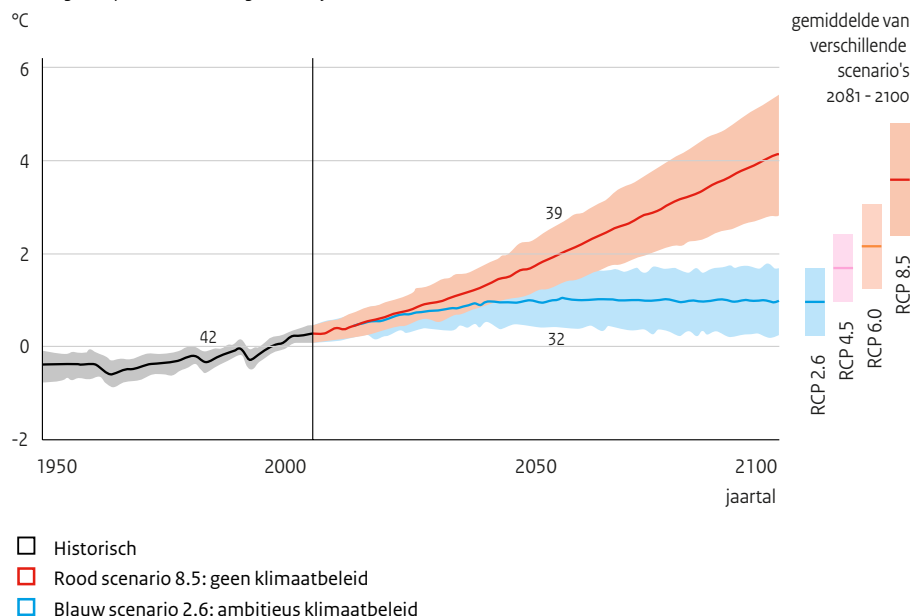
Figuur 1 Wereldgemiddelde oppervlaktetemperatuursverandering
